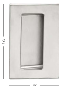
posuvné dveře D
